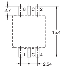
端子型3×3
